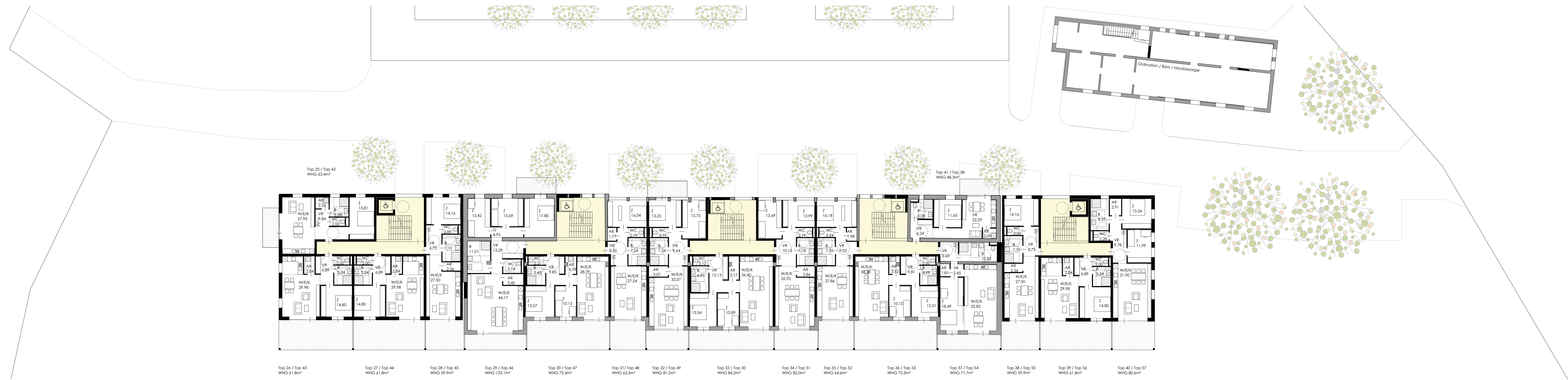
regelgeschoss | m 1:200
