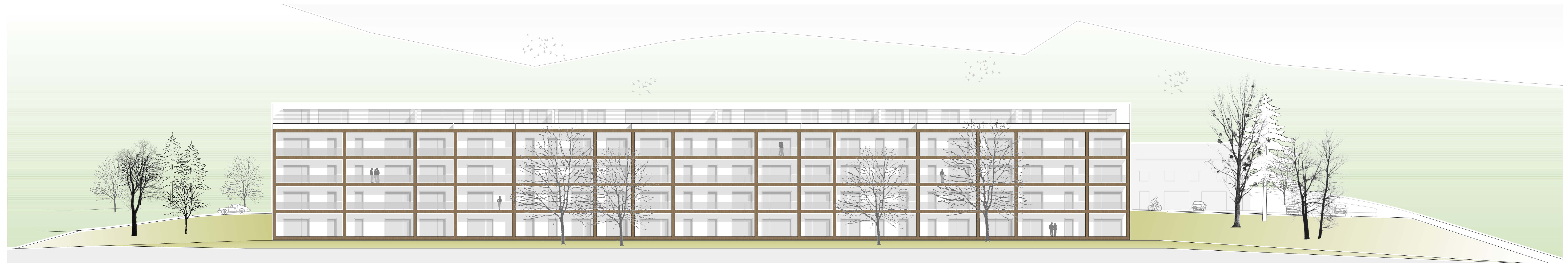
südansicht | m 1:200
