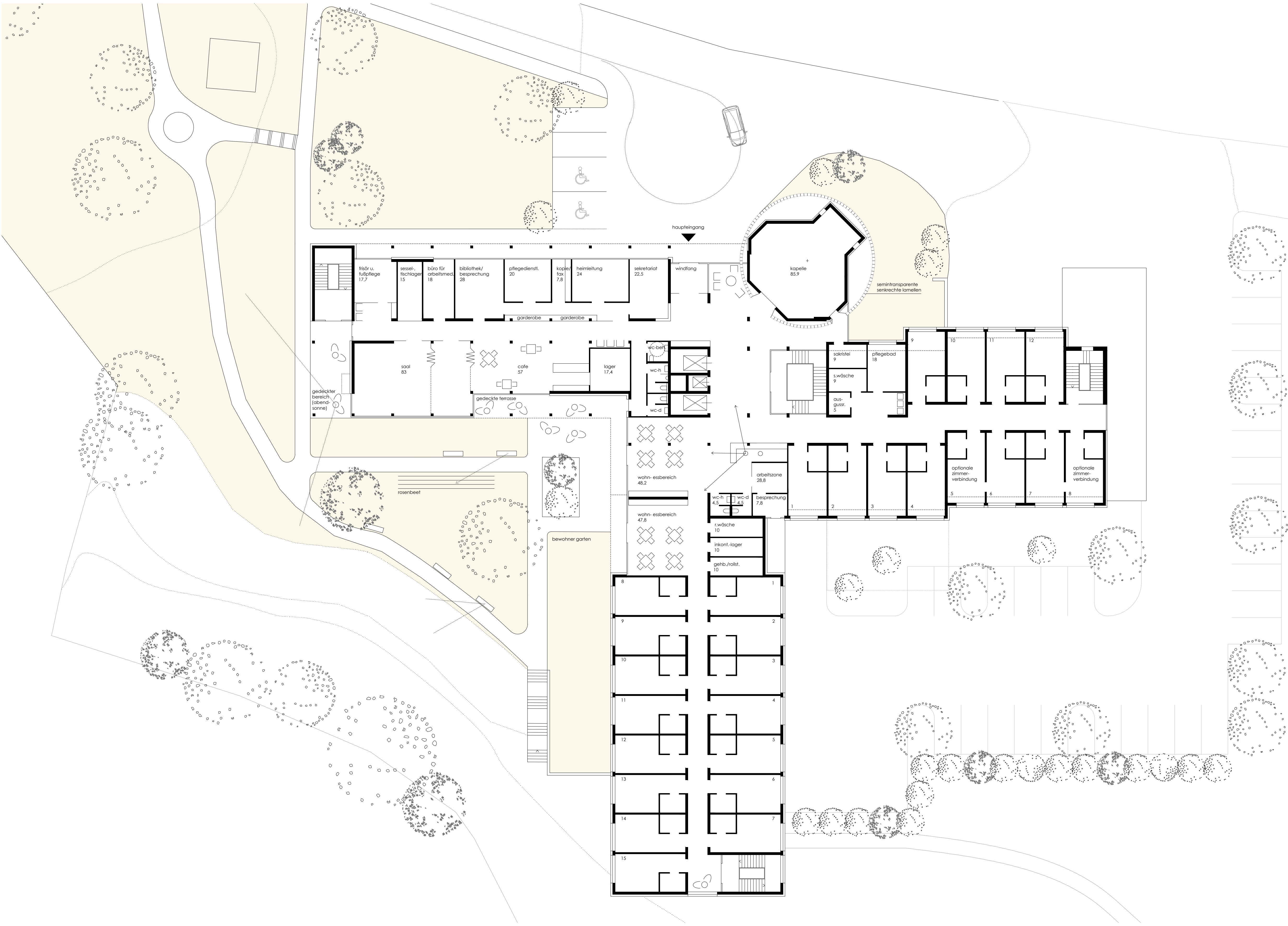
grundriss erdgeschoss
