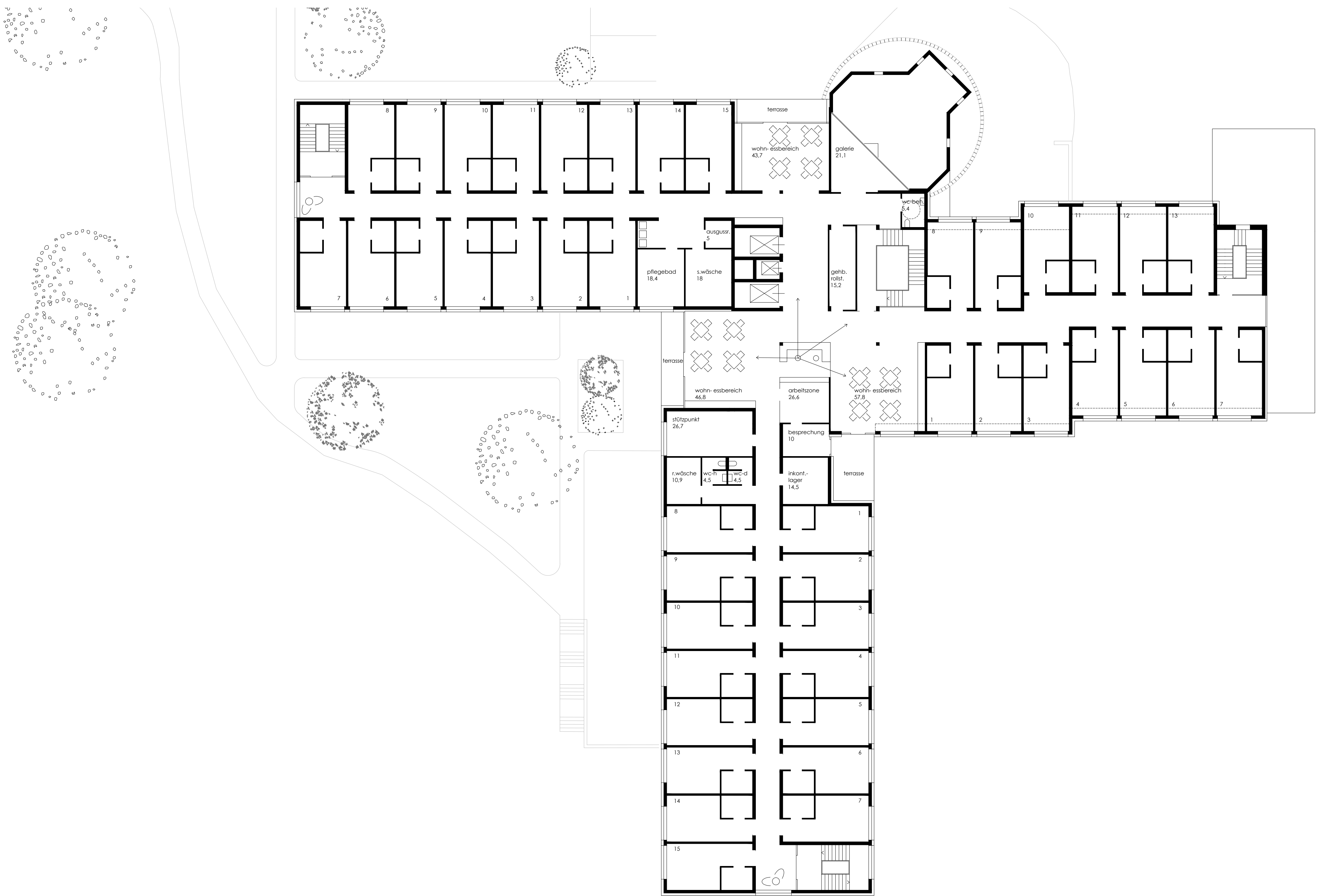
grundriss erdgeschoss
