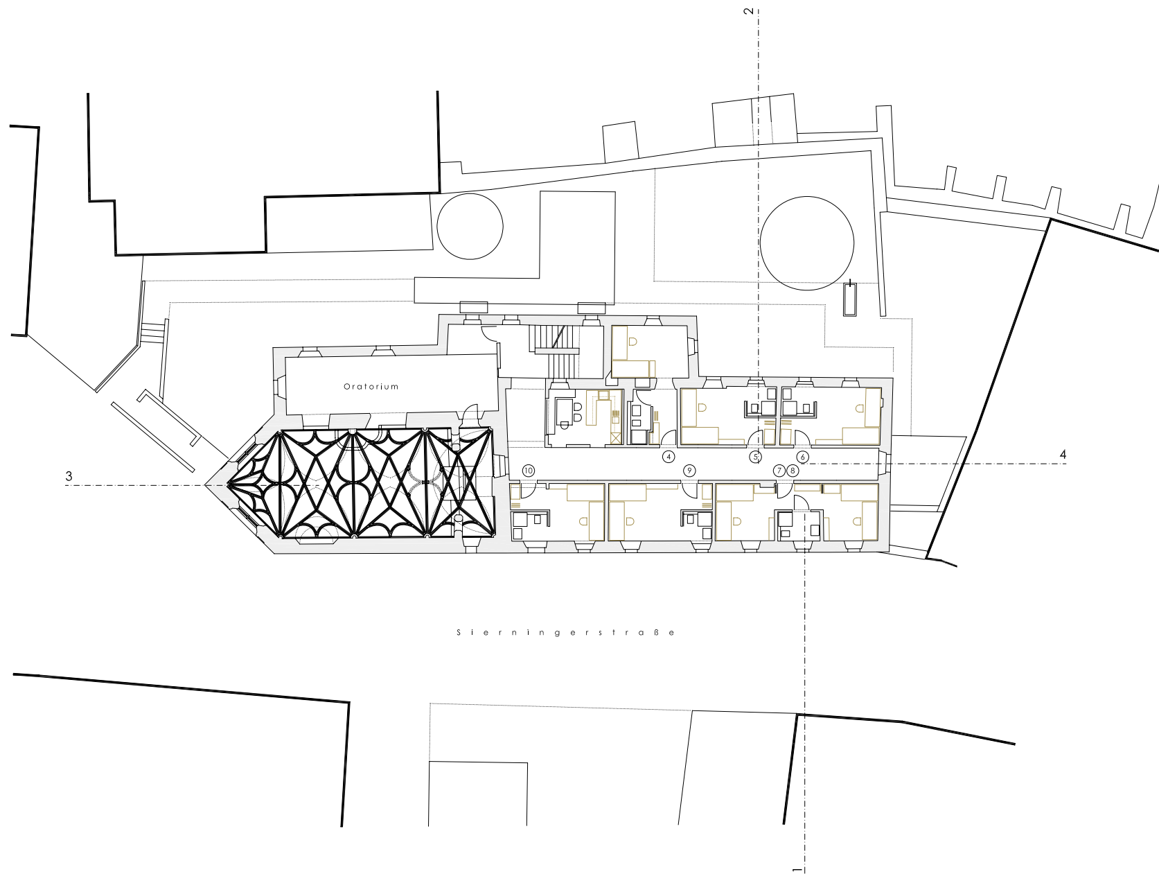
Obergeschoss
